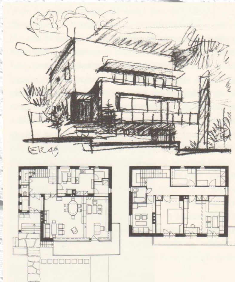
SKICA VILY EUGENA KRAMÁRA V BRATISLAVĚ, 1949
